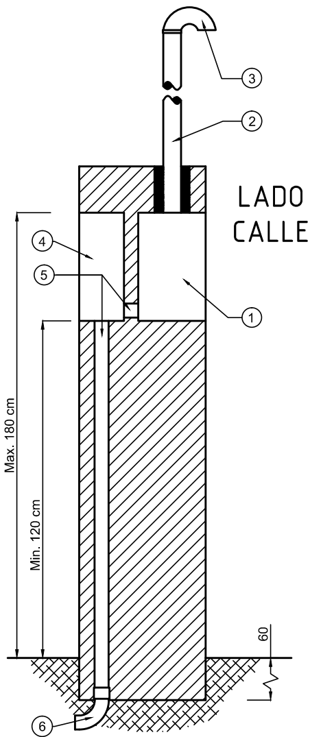
VISTA LAT. IZQ. DE CORTE CENTRAL
